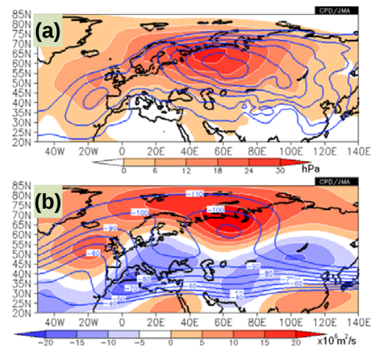
図7 2012 年 1 月 16 日～2 月 14 日平均 (a) 海面気圧、(b) 300hPa 流線関数 陰影は平年偏差。等値線は (a) 1020hPa 以上を 5hPa 間隔で、(b) -40 \times 10^6 \text{ m}^2/\text{s} 以下を 10 \times 10^6 \text{ m}^2/\text{s} 間隔で表示。
