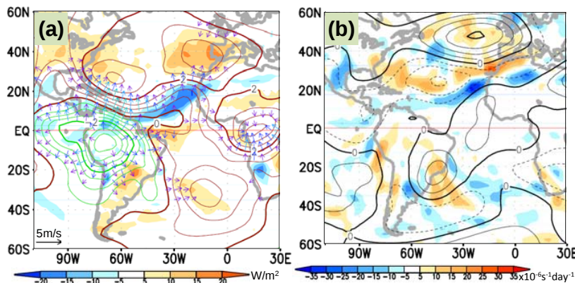
図 12 2011/2012 年冬平均 (a) 200hPa 速度ポテンシャル平 年偏差 (等値線)、200hPa 発散 風年偏差 (矢印)、及び外向き 長波放射 (OLR) 年偏差 (陰影)、 (b) 200hPa ロスビー波ソース (陰 影) 及び 200hPa 流線関数年偏 差 (等値線) 等値線間隔は (a) 0.5 \times 10^6 \text{ m}^2/\text{s} 、 (b) 3 \times 10^6 \text{ m}^2/\text{s} 。
