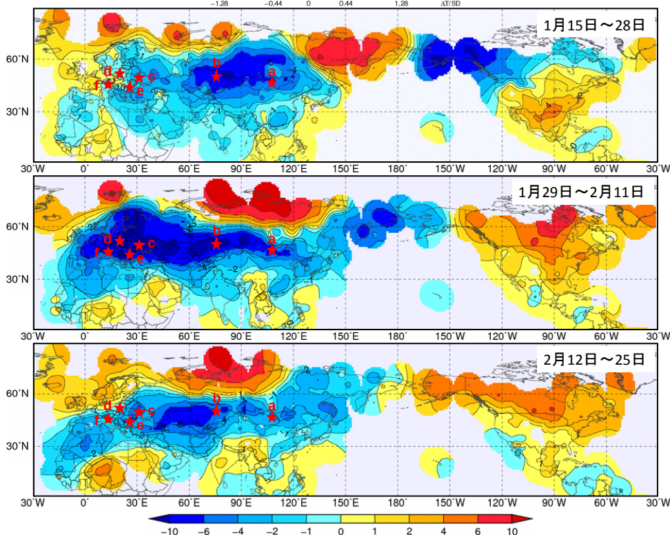
図 2 2012 年 1 月 15 日から 2 月 25 日の 2 週ごとの気温平年差 (°C) 各国から通報データによる。図中の星印 (a～f) は以下の地点 (国名) の位置を示す。 a: ウランバートル (モンゴル)、b: アスタナ (カザフスタン)、c: キエフ (ウクライナ)、d: ワルシャワ (ポーランド)、e: ブカレスト (ルーマニア)、f: トリエステ (イタリア)
