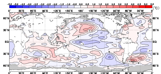
図6 2011/2012 年冬平均海面水温平年偏差
