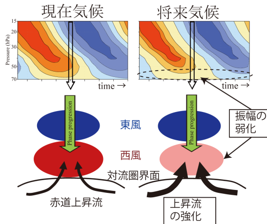
図2. 現在気候と将来気候における(上)東西風の時間-高度断面図と(下)QBOと赤道域上昇流の模式図。温暖化にともなって赤道域上昇流が強まり、下部成層圏最下層でのQBO振幅が弱まる事を示す。
